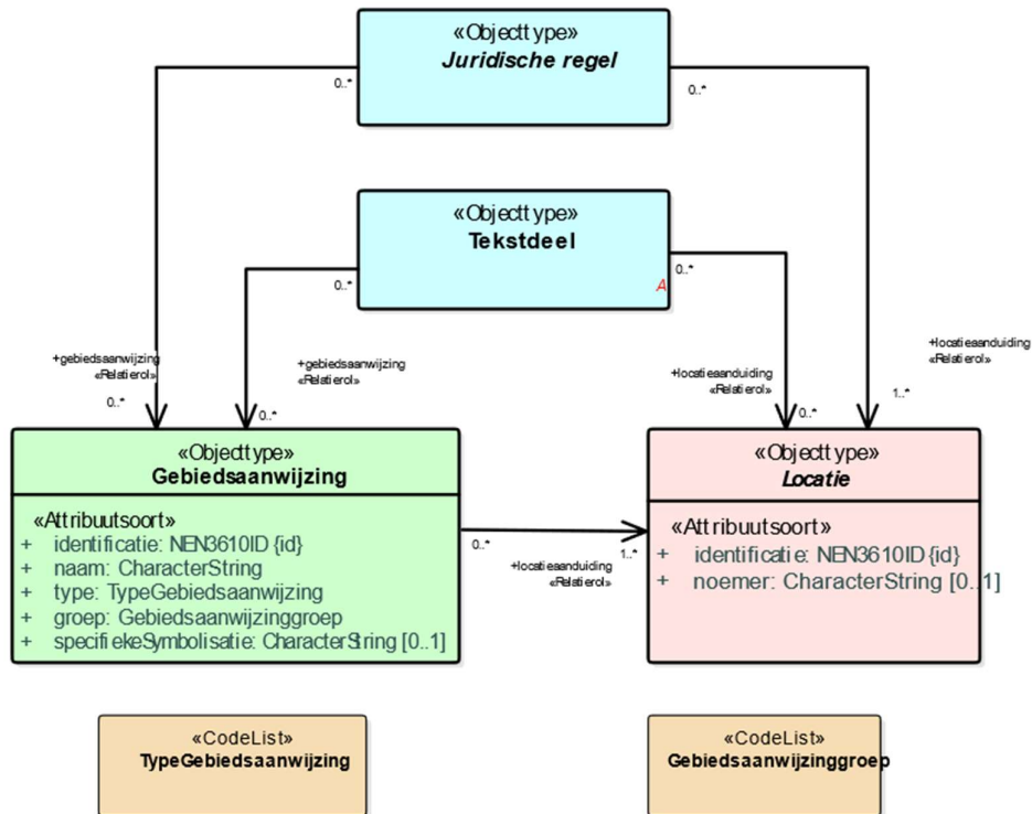
Figuur 41 Uitsnede uit IMOW-diagram voor objecttype Gebiedsaanwijzing
