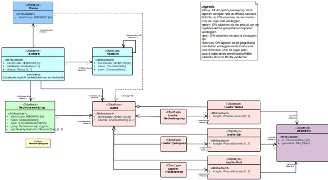
Figuur 12 UML-klassediagram van IMOW toegepast op het projectbesluit
