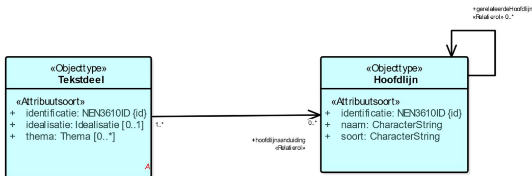
Figuur 17 Uitsnede uit IMOW-diagram voor objecttype Hoofdlijn
