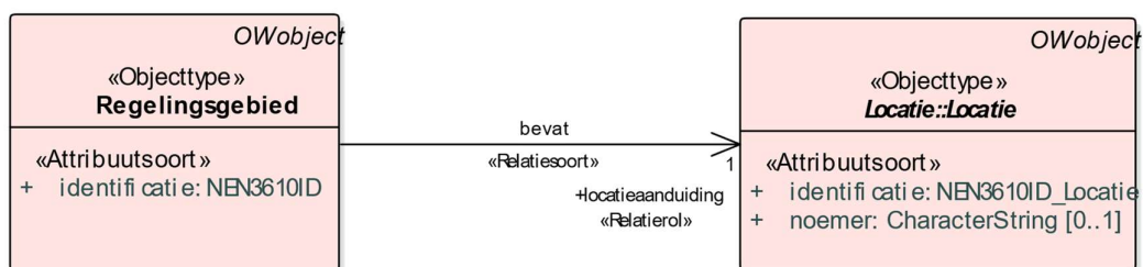
Figuur 21 Uitsnede uit IMOW-diagram voor objecttype Regelingsgebied
