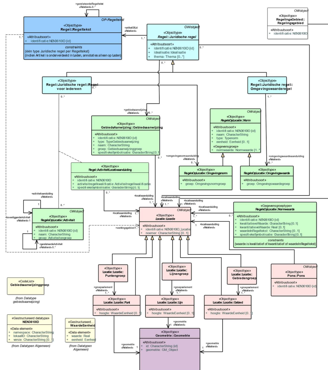
Figuur 25 UML-klassediagram van IMOW toegepast op het omgevingsplan
