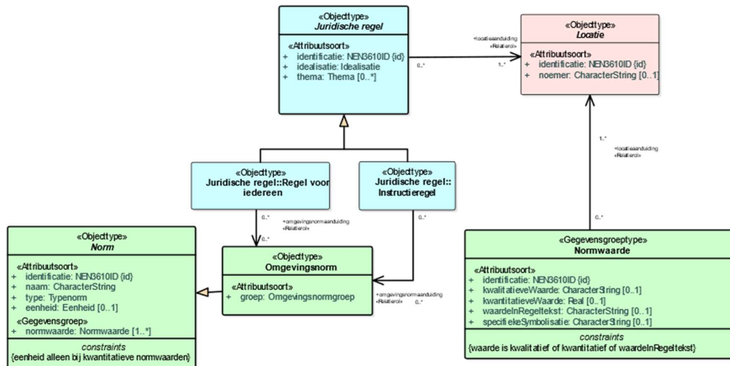
Figuur 40 Uitsnede uit IMOW-diagram voor objecttype Omgevingsnorm
