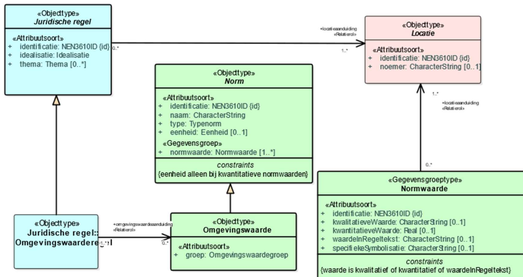
Figuur 37 Uitsnede uit IMOW-diagram voor objecttype Omgevingswaarde
