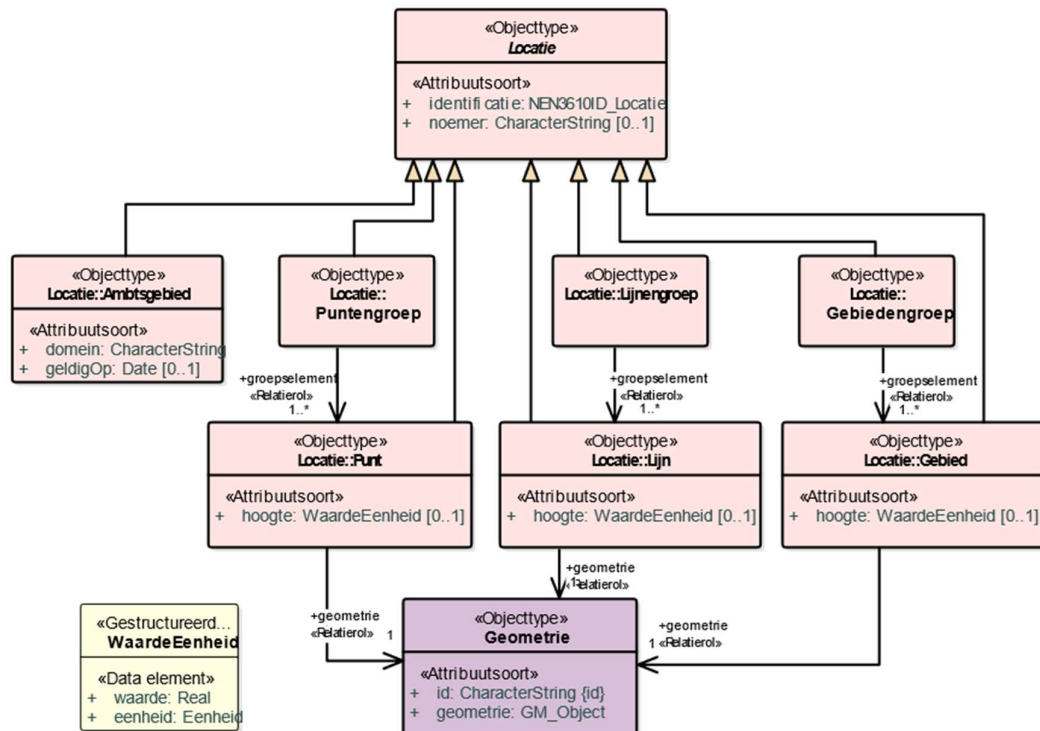
Figuur 33 Uitsnede uit IMOW-diagram voor objecttype Locatie
