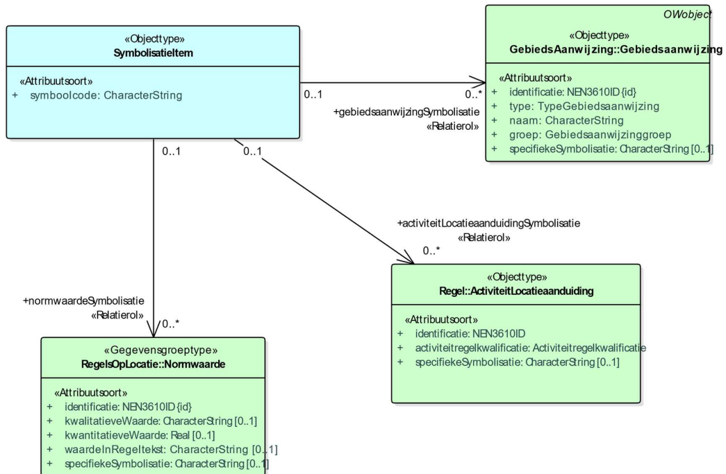
Figuur 45 Uitsnede uit IMOW-diagram voor objecttype SymbolisatieItem
