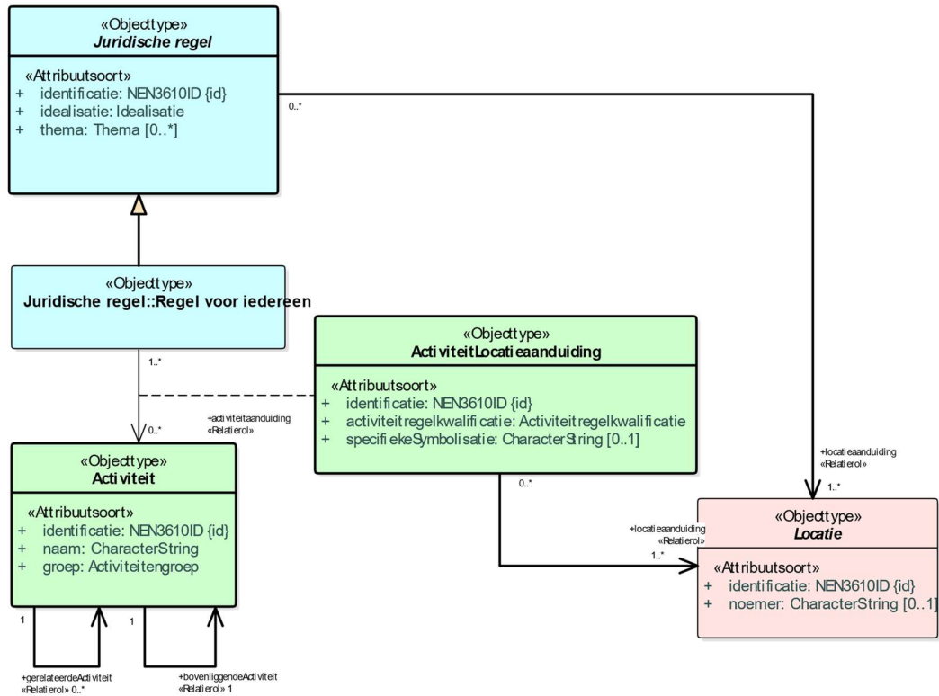
Figuur 35 Uitsnede uit IMOW-diagram voor objecttype Activiteit
