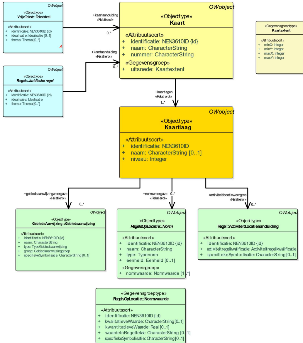
Figuur 43 Uitsnede uit IMOW-diagram voor objecttype Kaart
